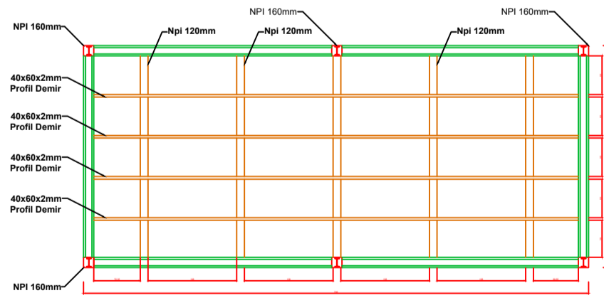
Üstten Görünüş (Çatı)
