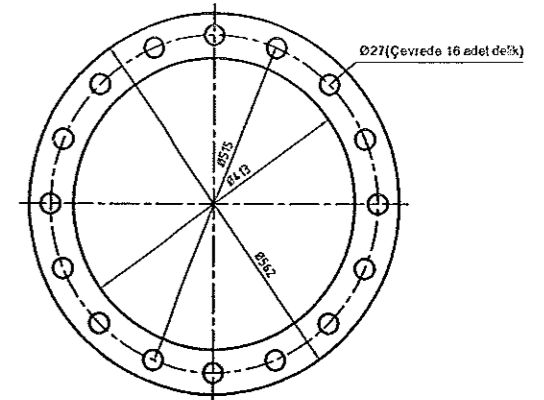
Ø5500 Kule Difüzörü Flaş Contası Resim No : 2.08.01781 - Poz :58 Kalınlık : 3 mm Malzeme : Kİngrit Miktar : .....7.....
