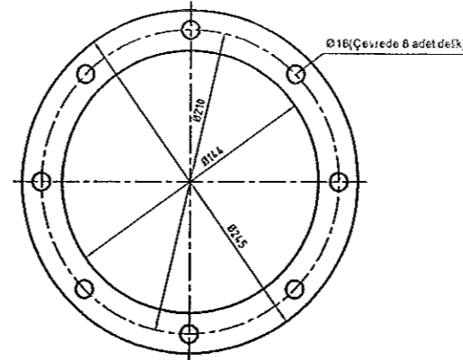
Ø5500 Kule Difüzörü Flaş Contası Resim No : 2.08.01781 - Poz :61 Kalınlık : 3 mm Malzeme : Kİngrit Miktar : .....8.....
