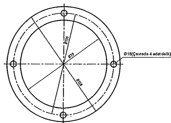
Ø5500 Kule Difüzörü Flaş Contası Resim No : 2.08.01781 - Poz :64 Kalınlık : 3 mm Malzeme : Kİngrit Miktar : .....36.....
