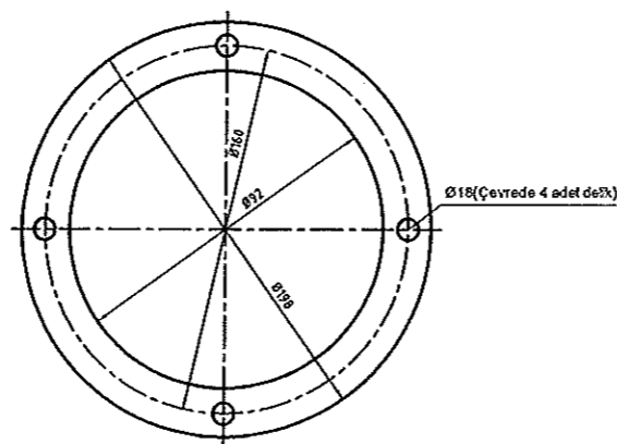
Ø5500 Kule Difüzörü Flaş Contası Resim No : 2.08.01781 - Poz :63 Kalınlık : 3 mm Malzeme : Kİngrit Miktar : .....1.....
