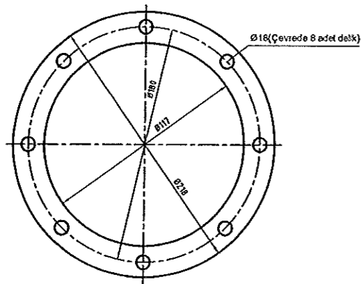
Ø5500 Kule Difüzörü Flaş Contası Resim No : 2.08.01781 - Poz :62 Kalınlık : 3 mm Malzeme : Kİngrit Miktar : .....7,5.....
