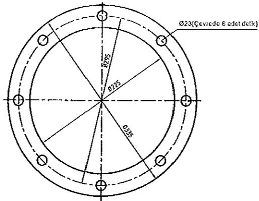
Ø5500 Kule Difüzörü Flaş Contası Resim No : 2.08.01781 - Poz :60 Kalınlık : 3 mm Malzeme : Kİngrit Miktar : .....4.....
