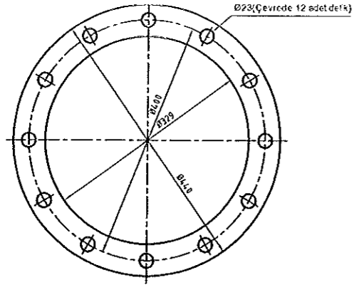
Ø5500 Kule Difüzörü Flaş Contası Resim No : 2.08.01781 - Poz :59 Kalınlık : 3 mm Malzeme : Kİngrit Miktar : .....2.....
